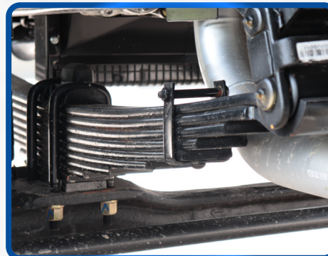
Nhíp trước 11 lá, giảm chấn thủy lực
